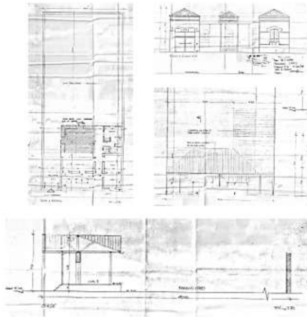
Planos de planta, fachada principal, panta de cubiertas y corte transversal, presentados con el proyecto de intervención presentado ante la Junta de Protección de Patrimonio Urbano en 1998.
